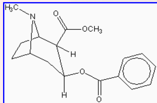
Cocaïne
